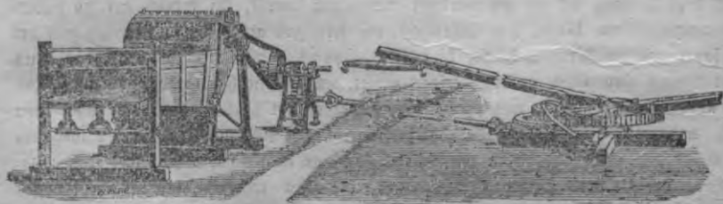
(Kauschenbacha pahrlabotā stiftu kulamā maschine.)
