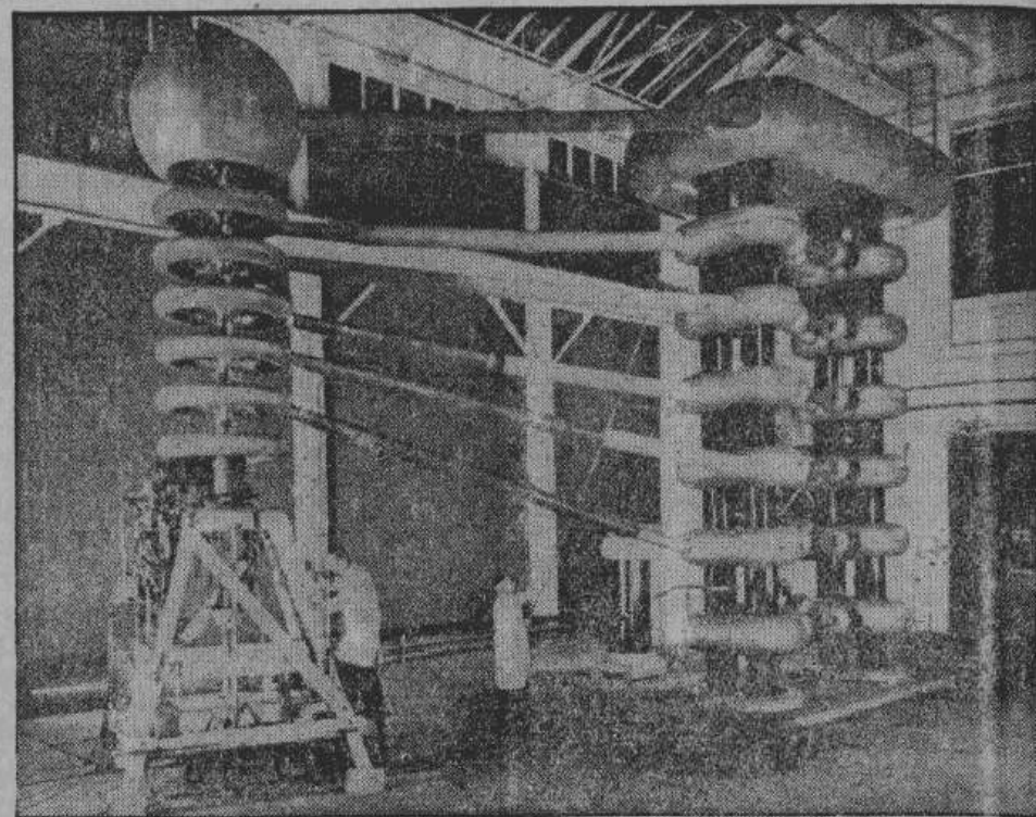
Величайшее и сильнейшее рентгено-терапевтическое оборудование, имеющее напряжение в один миллион вольт. Предназначается для специальных способов лечения в Берлине.
