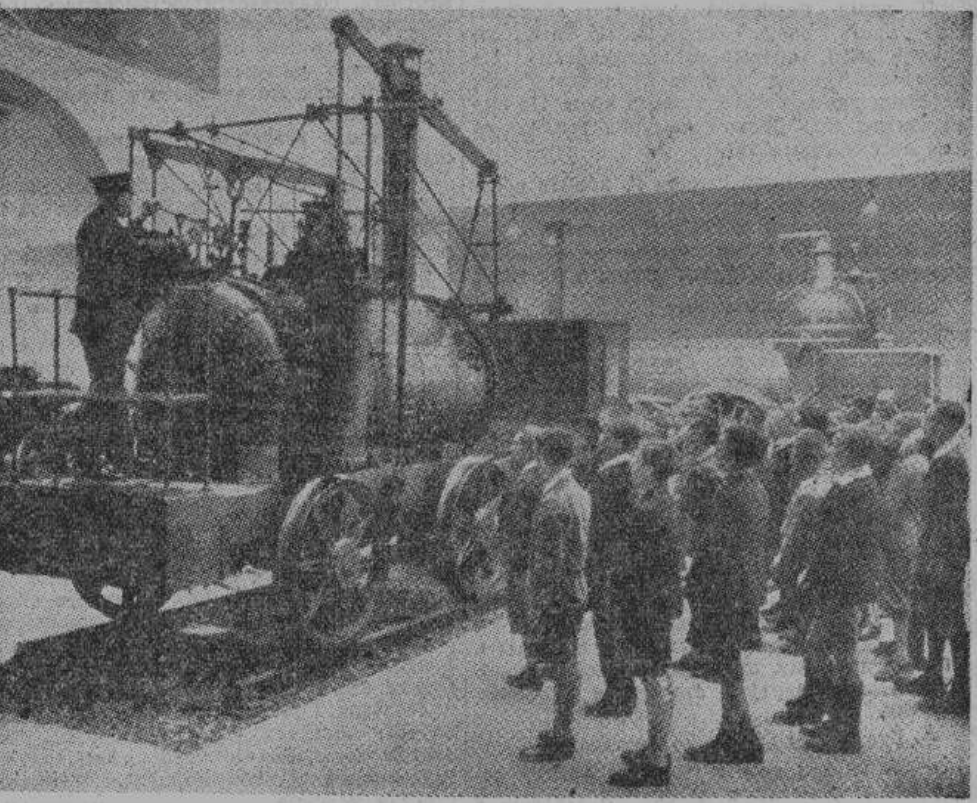
Точная копия первого локомотива, построенного в 1813 году.
