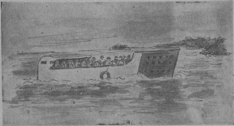
Английское судно для высадки войск. Носовая часть откидывается вперед и при высадке с судна служит трапом. Судно способно вместить один танк и сорок солдат.
