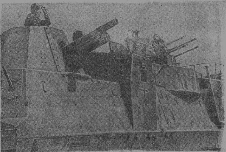
Германский бронепоезд в этой войне сильно отличается от бронепоездов первой мировой войны. Помимо общетехнических усовершенствований и усиления боевых качеств, нынешний бронепоезд снабжен сильной противовоздушной артиллерией.
