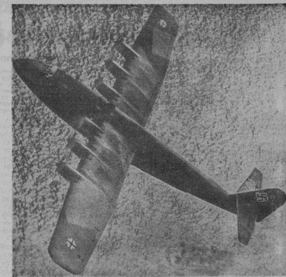
«Викинг ВВ 222» — крупнейшая авиалодка германского военно-воздушного флота. Этот гигантский гидросамолет оборудован шестью моторами, длина его корпуса составляет 37 метров, а высота 5,6. Размах крыльев — 46 метров. В двухэтажных внутренних помещениях самолета легко помещаются сто солдат, со всем вооружением или же соответствующее количество груза. Гидросамолет вооружен сильной артиллерией и пулеметами.
