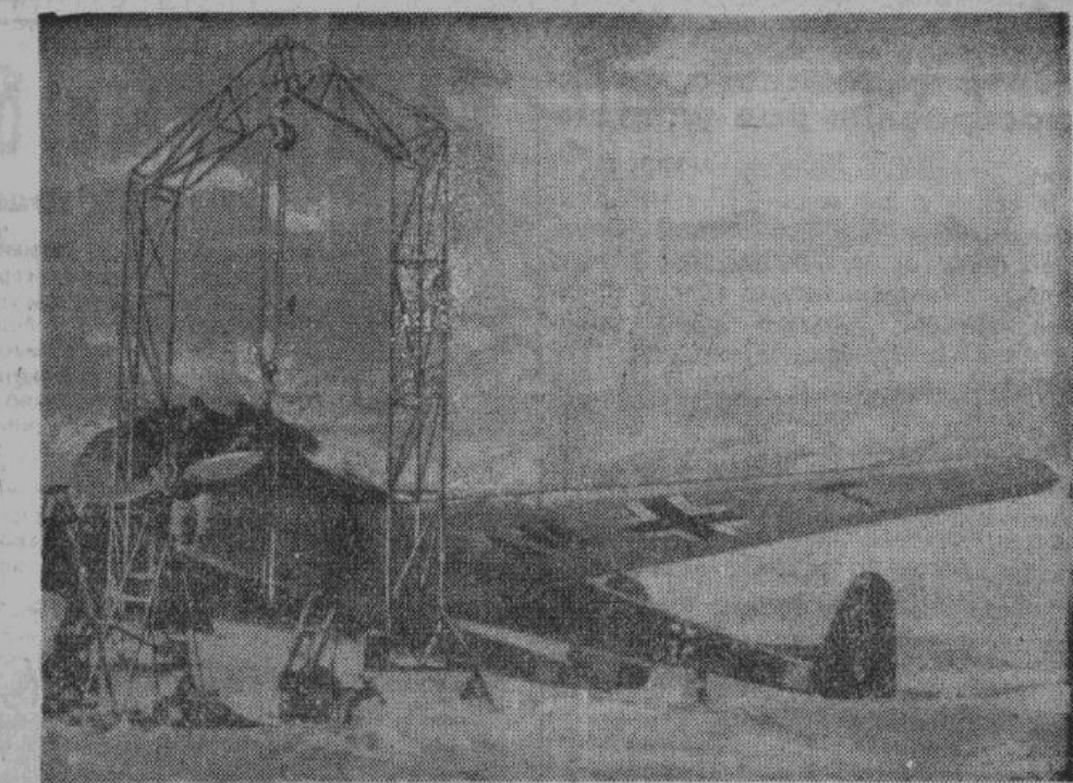
Германские аэродромы на дальнем севере оборудованы первоклассными мастерскими, производящими любой ремонт самолетов. На снимке — моторы германского разведчика заменяются с помощью специального передвижного крана.
