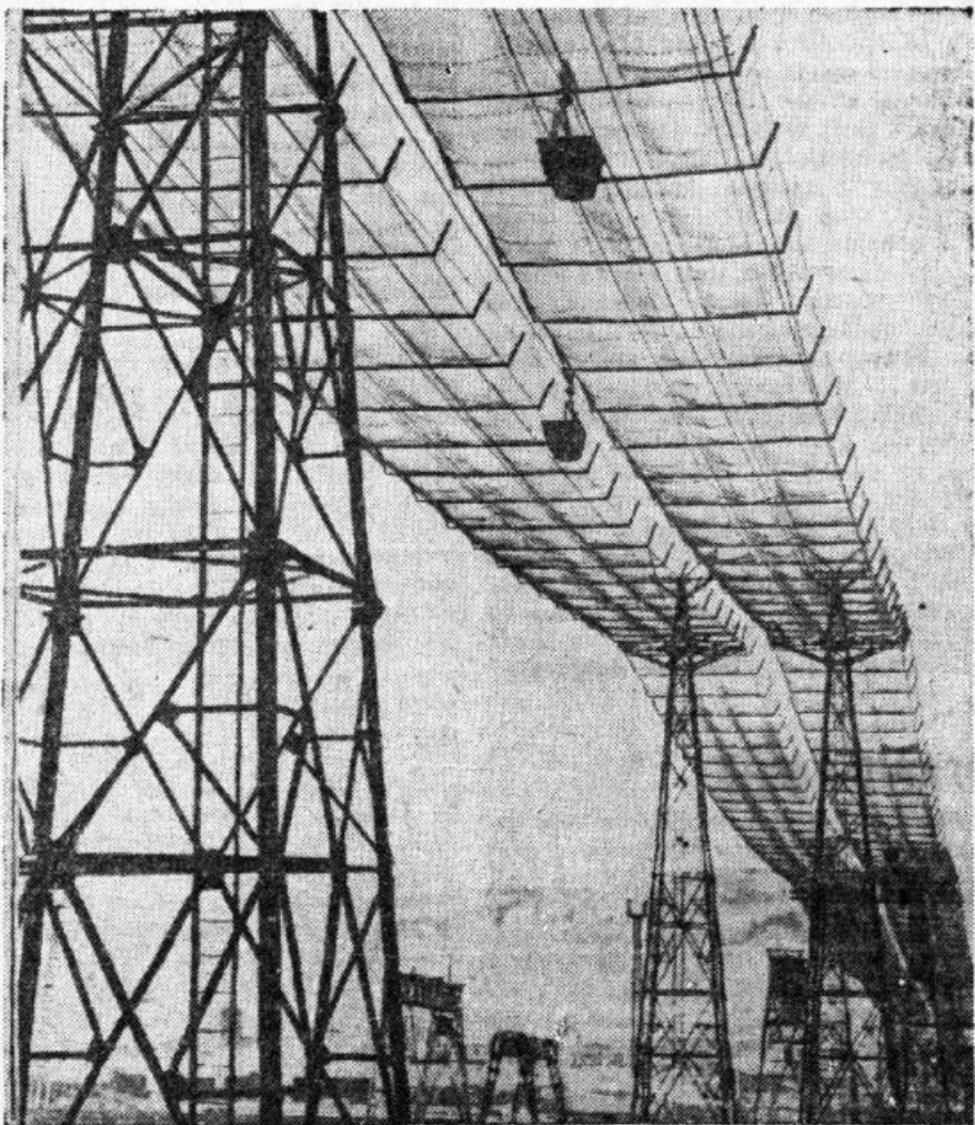
Lai materiālu transportēšanu Kuibīševas hidroelektrostacijas celtniecībā darītu ērtāku, pāri Volgai izbūvēts tauvu ceļš. Tauvu ceļa vagonetes no Volgas labā krasta uz kreiso pārvadās akmeņus un šķembas, bet pretējā virzienā — smiltis betona ražošanai.
