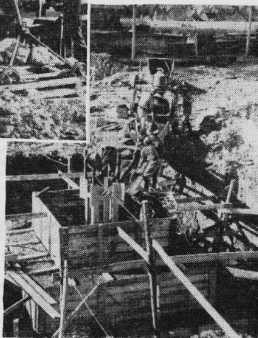
Attēlā: grunts izsmelšanā masta pamatu betonētāji ar lābiem panākumiem izmanto, lūk, šo celtni (augšējais attēls), kas ne tikai atvieglo darbu, bet arī izveido valrākus cilvēkus. Sprāgst (apakšējais attēls) masta balstu betonēšana.
