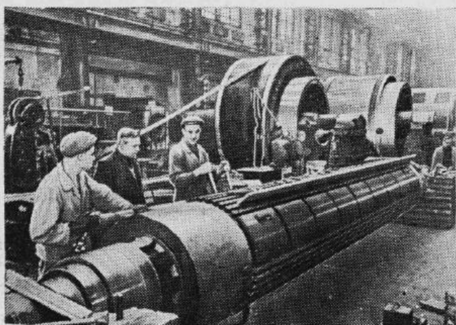
Attēlā: 100 tūkstoš kilovatu lielā turboģeneratora sakniedšana. (No kreisās) kniedētājs N. A. Orlovs, vecākais meistars G. A. Kulīcevs un kniedētājs V. I. Samorukovs.
