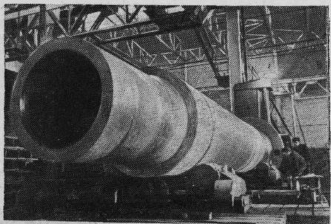
Leningrada. S. Kļova vārdā nosauktajā rūpnīcā „Elektrosila”, izgatavo spēcīgus turboģeneratorus ar 150 tūkstoškilovatu jaudu. Uzņēmumā: virpotājs G. Butusovs apstrādā turbīnas rotoru.
