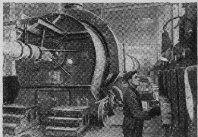
Attēlā: Spaskas cementa rūpnīcas apdedzināšanas cehs. Pie vadības pulst rotējošās krāsns labākais mašīnists b. J. Sistērovs, kurš maigās uzdevumu izpilda par 106 procentiem. TASS fotochronika
