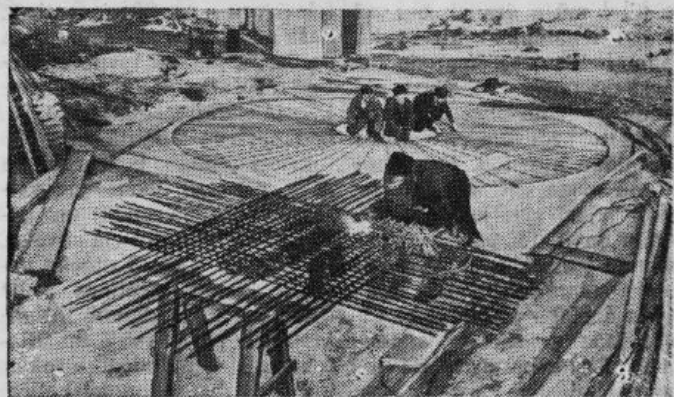
Attēls: stiegrotāja brigade pagatavo jaunās centralās elektrostacijas dūmeņu stiegrojumu.
