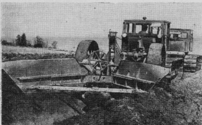
Attēlā: mechanizatori Slavinskis un Šņacis ar traktoriem S-80 un jauno arklu LKA-2 dzen vajējos grāvjus.
