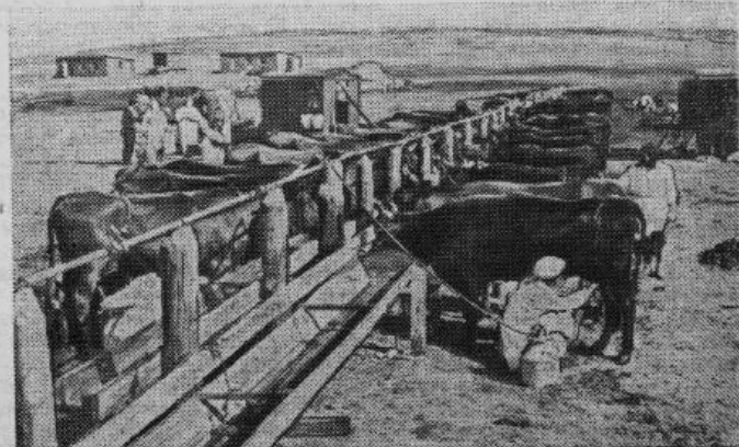
Attēlā: padomju saimniecības № 3 pārvietojamā mehaniskā slaukšanas līce.
