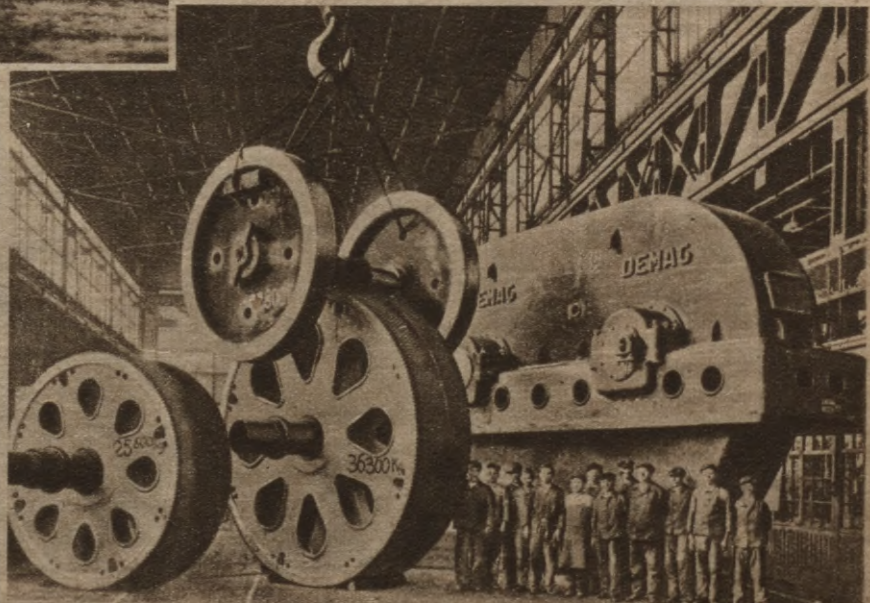
150.000 kg sver šie dzelzs veltuves zobrati.
