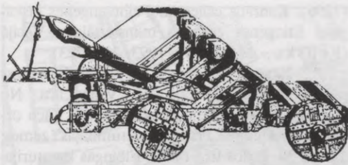
Akmeņu metamā mašina. Pēc Rūdolda Emsa «Pasaules hronikas 1383» zīmējuma (Mench, Leibling 1983, Abb. 48).
