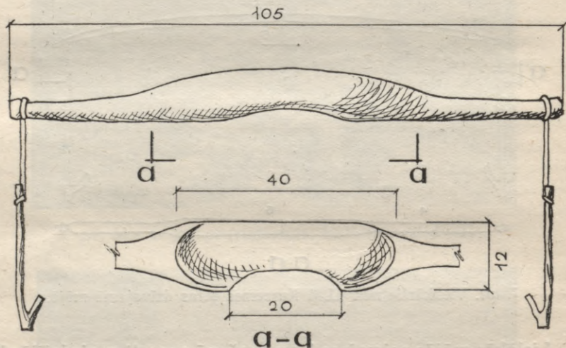
8. att. Izdobtie nēši LLM Kurzemes sētas dzīvojamā mājā.
