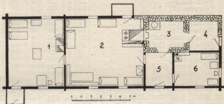
31. att. Dzīvojamās mājas plāns Talsu apr. Lībagu pag.
