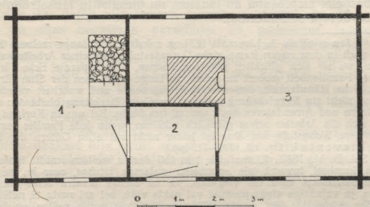
52. att. Plāns pirtij ar dzīvojamo kambari Valmieras apr. Sēļu pag. «Rūnās» (tagad LLM Vidzemes sētā).
