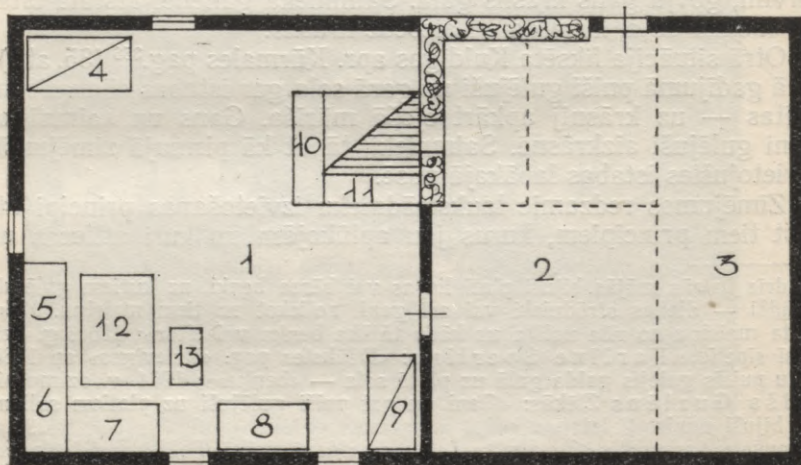
34. att. Dzīvojamās mājas plāns Kuldīgas apr. Lutriņu pag. «Skudrās» (VVM PV 3079. mape, 81. dok.).
