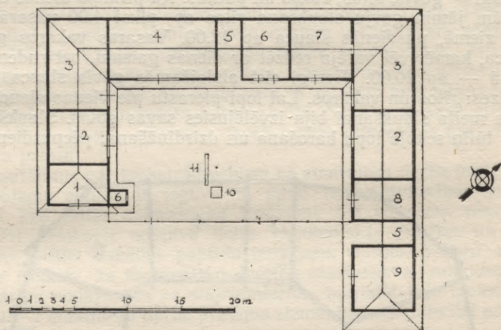
2. att. Pakavveida laidars Liepājas apr. Rucavas pag. «Dejos» (tagad LLM Kurzemes sētā).
