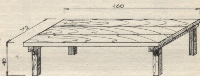
43. att. Lāviņa — «brička» Kuldīgas apr. Snēpeles, Turlavas, Raņķu, Skrundas pag. (VVM PV 3083. mape, XXIX dok.).
