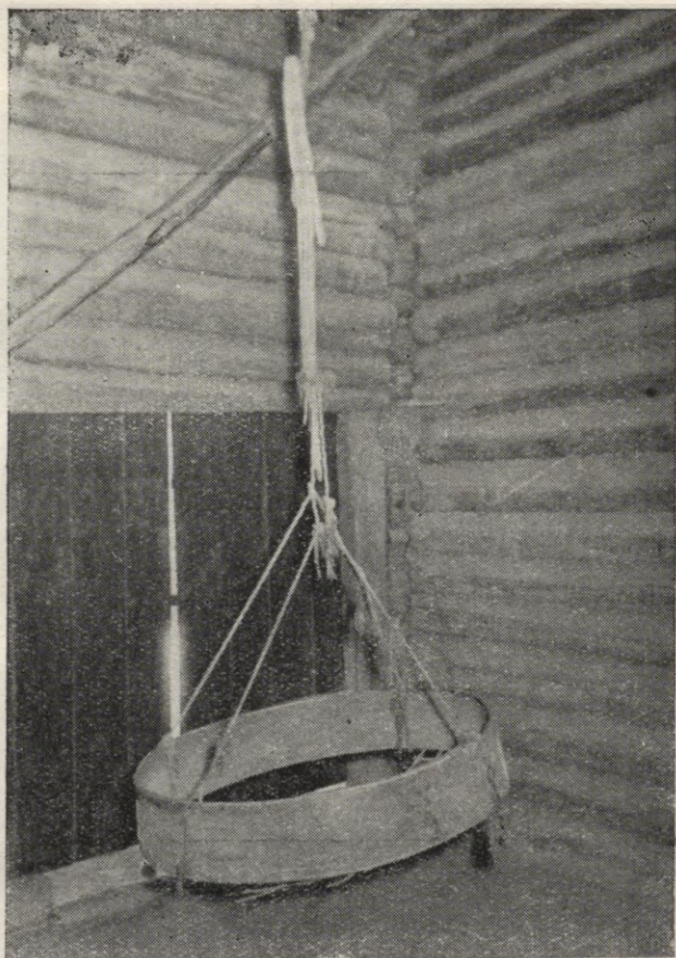
17. att. Kretuļa pakāršanas veids LLM Vidzemes sētas rijā.
