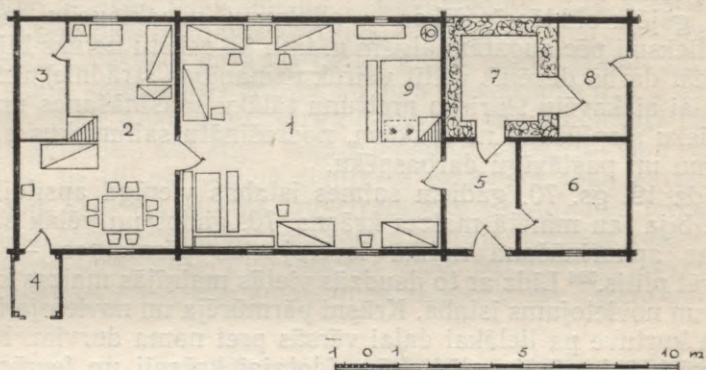
28. att. Dzīvojamās mājas plāns Talsu apr. Nurmuižas pag. Strēļos» (VVM PV 2948. mape, 301. dok.).
