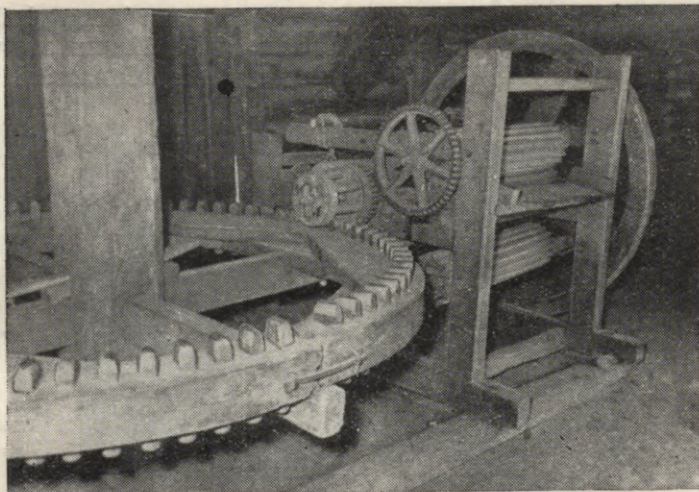
20. att. Ar zirgu darbināmā līnu maļamā mašīna LLM Zemgales sētas rijā.
