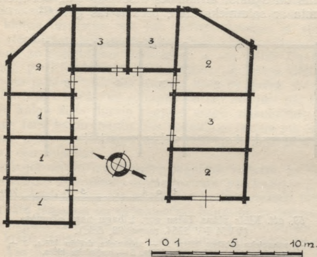
58. att. Kalpu rinka plāns Jelgavas apr. Sīpeles pag. «Poķos» (tagad LLM Zemgales sētā).
