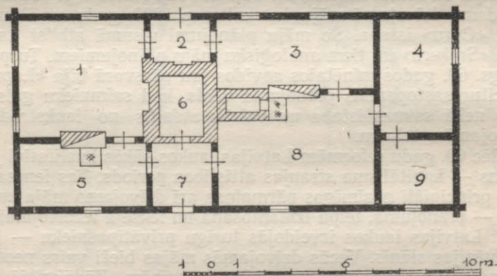
24. att. Dzīvojamās mājas plāns Bauskas raj. Bruknas c. p. «Lapušos».
