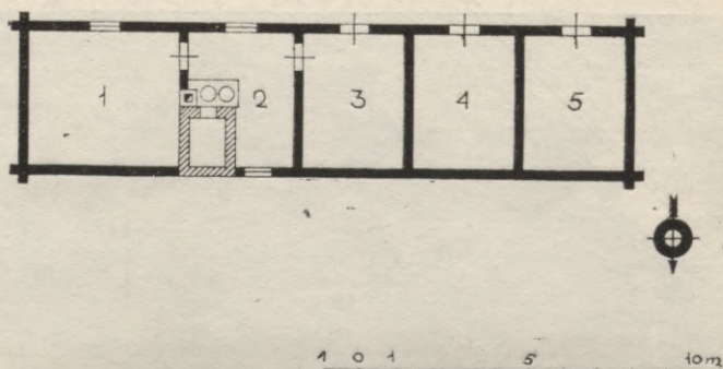
49. att. Kalpu dzīvojamās mājas plāns Bauskas raj. Ceraukstes c. p. «Ribās».
