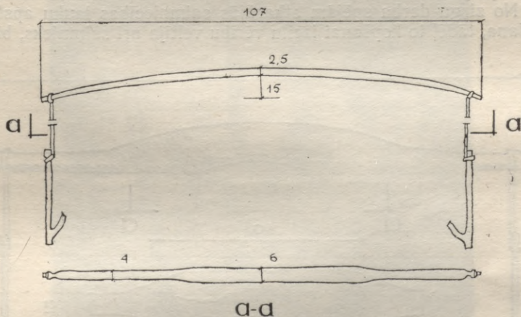
7. att. Vienkāršie nēsi LLM Kurzemes sētas dzīvojamā mājā.
