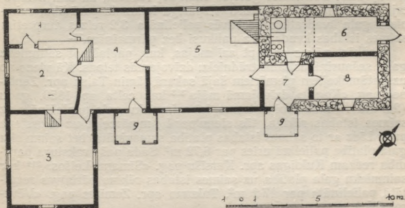
25. att. Dzīvojamās mājas plāns Talsu apr. Vandzenes pag «Muciniekos» (VVM PV 2948. mape, 245. dok.).
