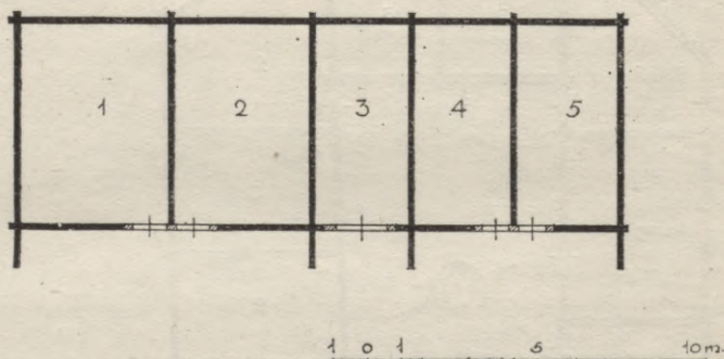
59. att. Klēts plāns Talsu apr. Lībagu pag. «Tomos» (VVM PV 2954. mape, 28. dok.).
