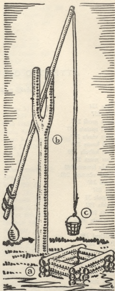
Vinda un aka a — akas grodi; b — vinda; c — akas spainis
