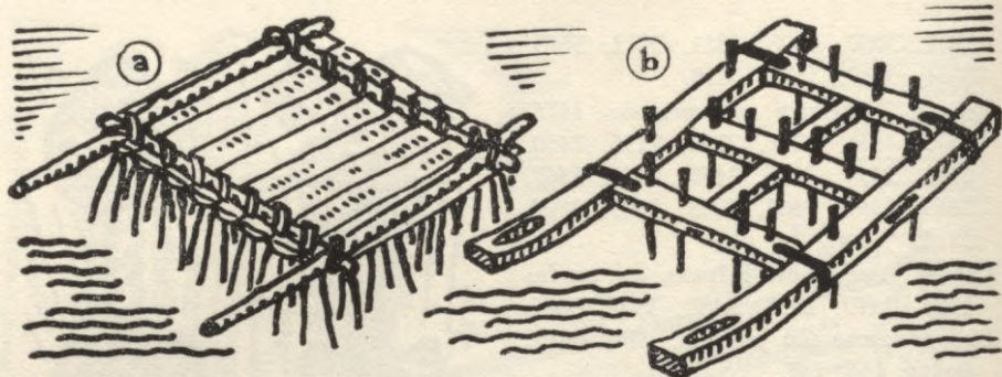
a — Koka ecēšas — egļi, gatavoti no šķeltām zarainām egļu galotnēm, sastiprinot tās vienu otrai blakus ar zariem uz leju; zarus atstāja apm. 40—50 cm gaļus; b — dzelzs tapu ecēšas
