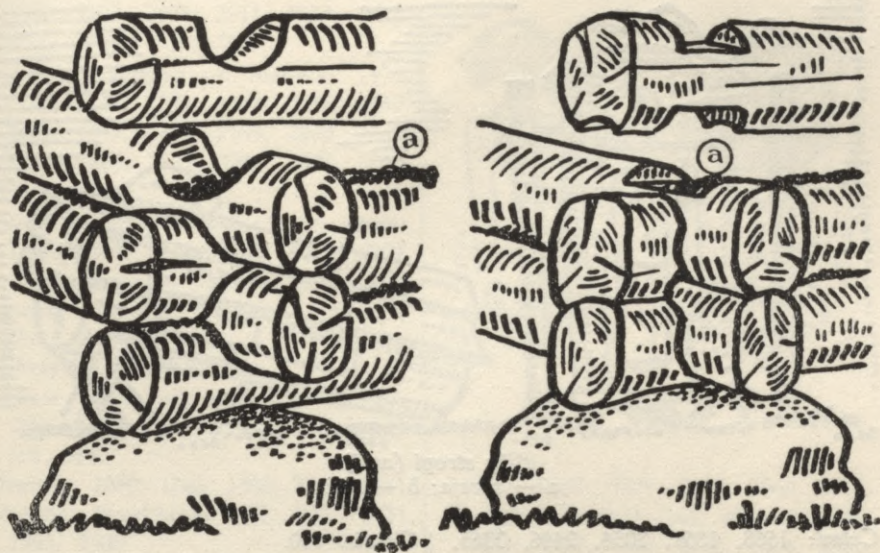
Baļku savienojumi pakšī a — sūnas
