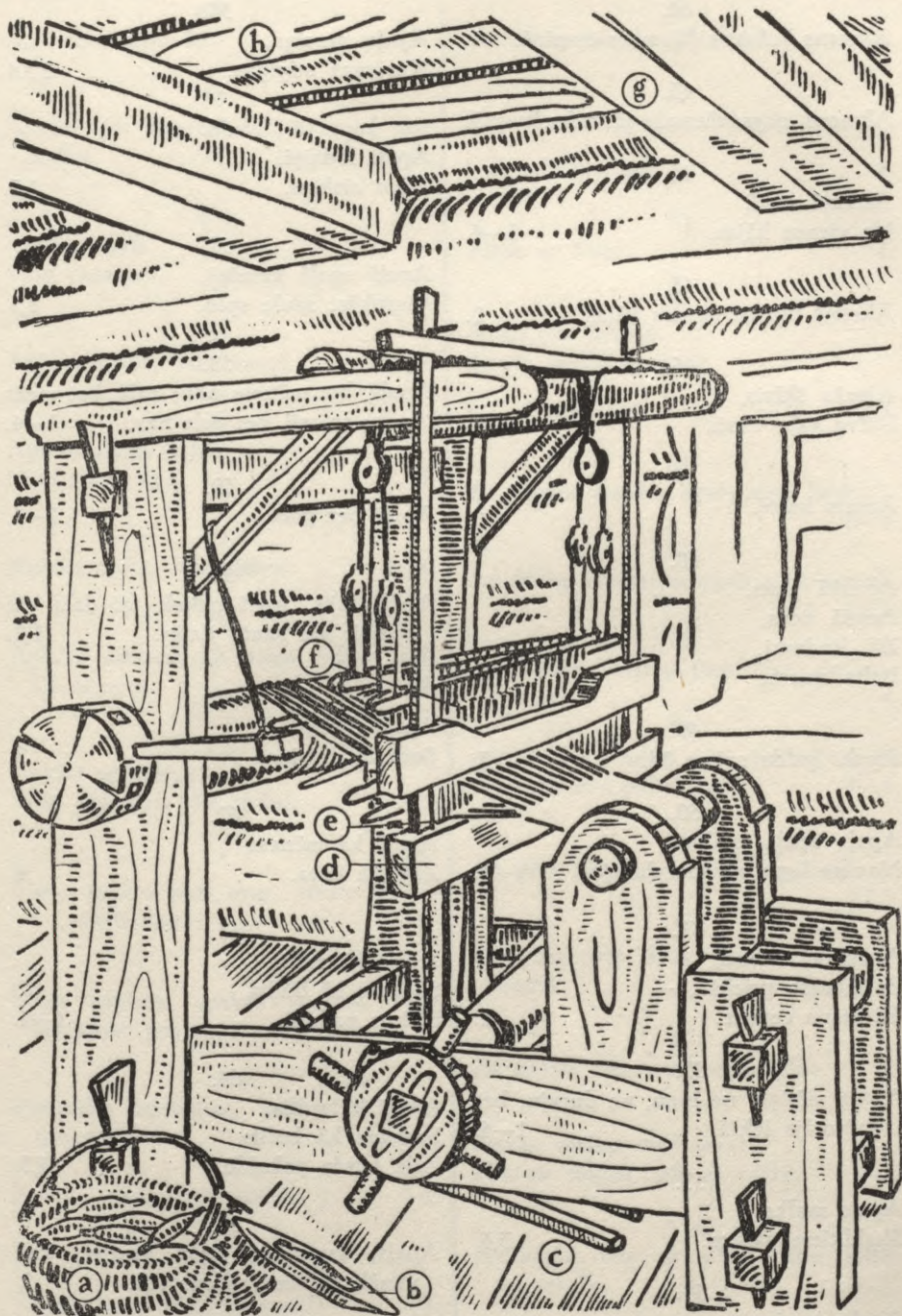
Aužamie stāvi (stelles)
