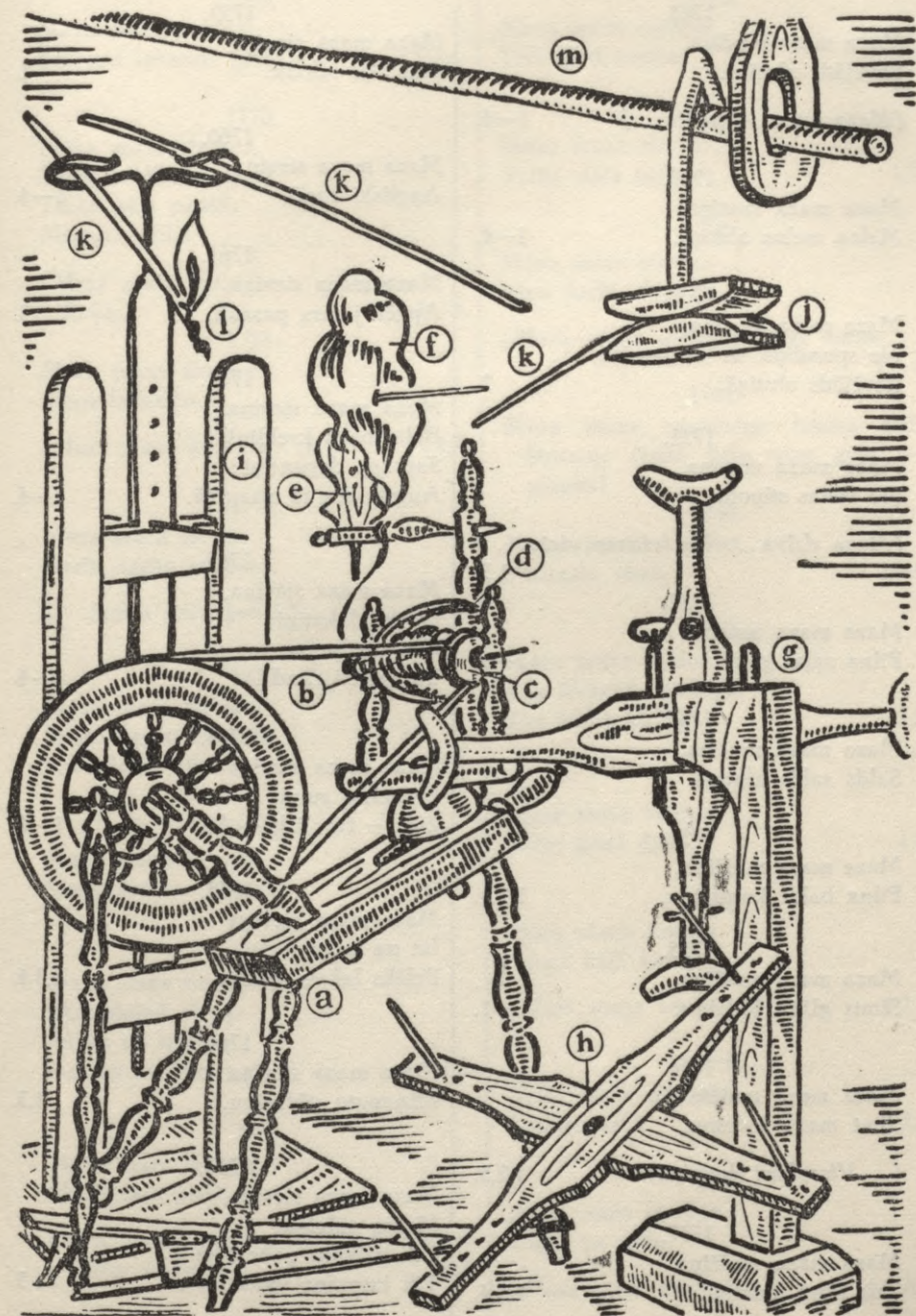
Vērpjamais ratiņš, fitavas un lāktuži a — ratiņš; b — ratiņa spole; c — ratiņa skriemelis; d — ratiņa spārns; e — sprēsliņa; f — kodeļa (ērkulis); g — fitavas; h — kluģi; i — lākturis; j — lākturis kāsi; k — skali; l — ogle; m — kārtiņa (parasti krāsns tuvumā)
