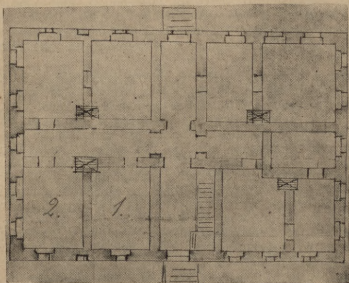
Rēzeknes apriņķa skūlas ākas pirmō stōva plans. Sastōdeits 1857. g. (1. — kanceleja, 2. — biblioteka, pōrējōs ustobas — skūlas pōrziņa dzeivūklis).
