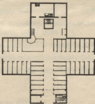
Ļaudonas baznīca, ap 1692. g. darinātais būvmets (plāns) R. V. u. S. B., baznīcas III, 12
