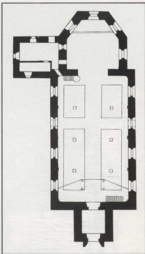
Iecavas baznīcas plāns. Uzmērojums, 1939. g.
