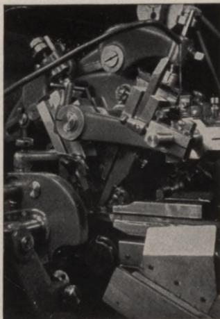
Skrūvju automats
