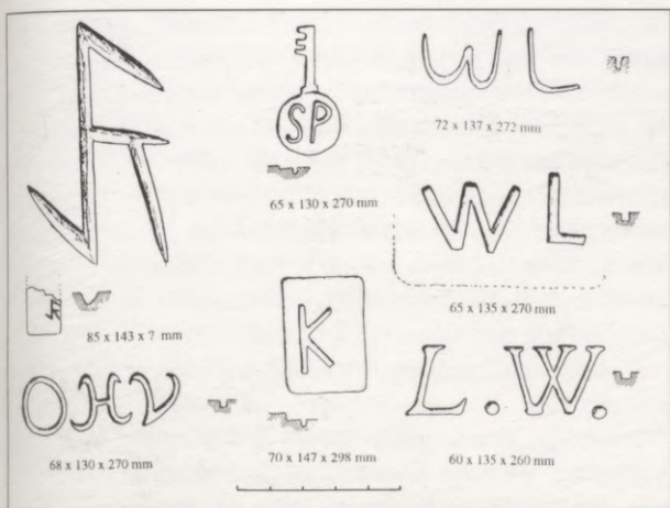
4.att. Melngalvju nama celtniecībā un vēlākās pārbūvēs lietoto ķieģeļu markas. Zīmējis arhitekts I.Dirveiks
