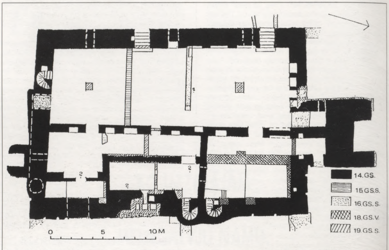
3.att. Melngalvju nama pagrabstāva plāns
