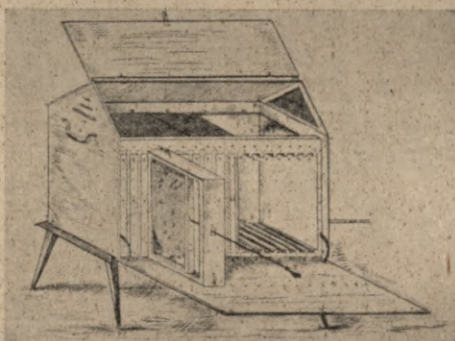
114. zīm. Munna strops.
