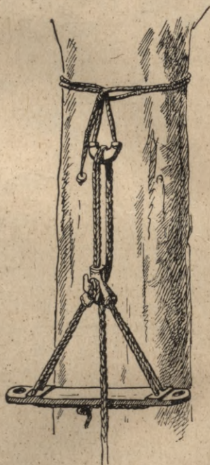
165. zīm. Kāpšanai uzkarināts dzeinis.
