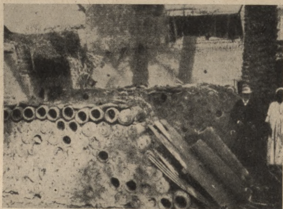
15-a att. Mūslaiku Ēģiptes drava.
