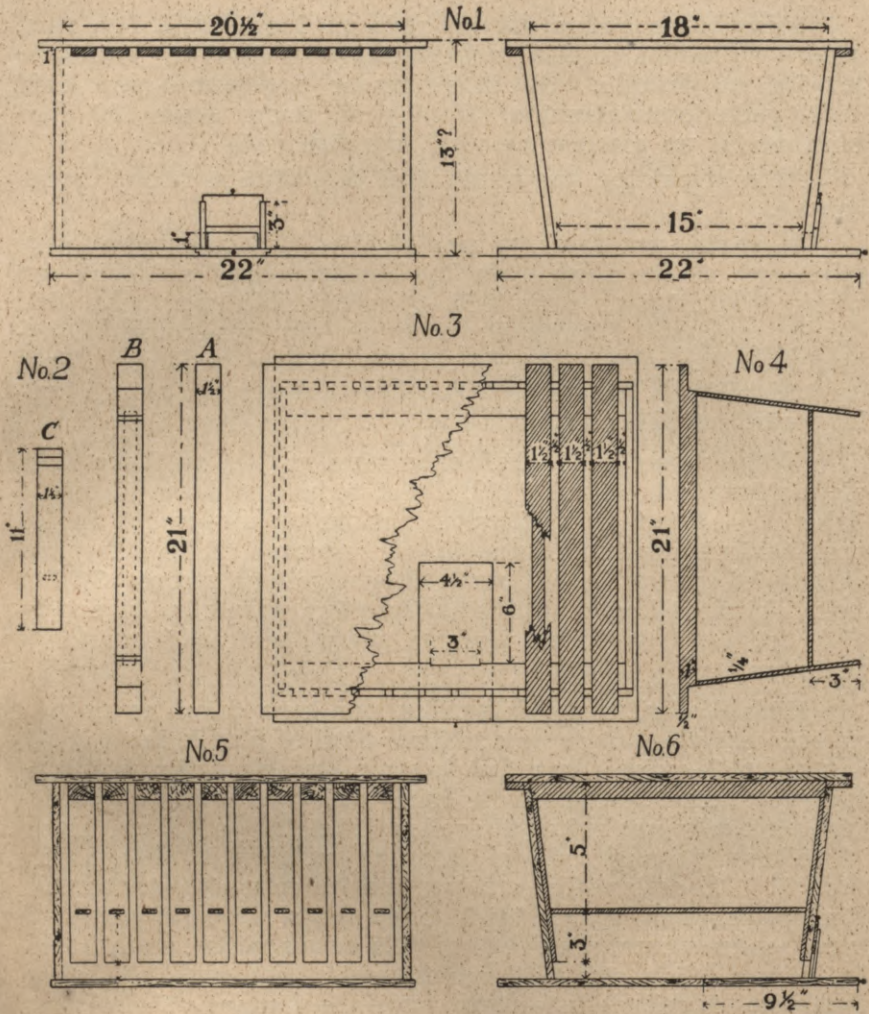
113. zīm. J. A. strops ar iekarināmiem rāmīšiem.
