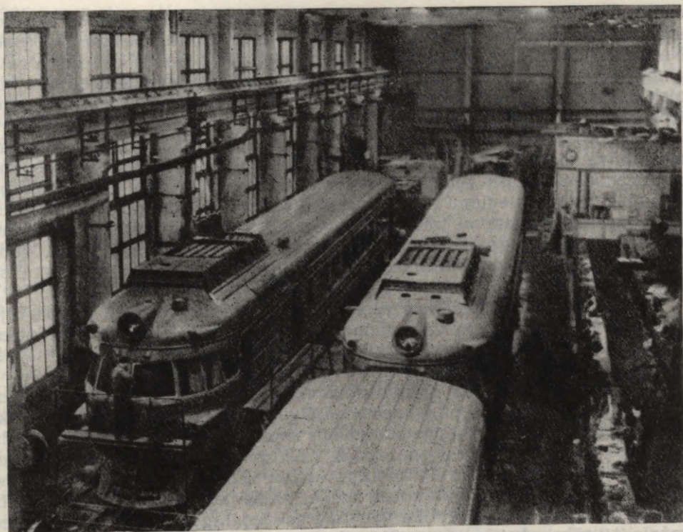
Rīgas vagonu rūpnīcas dizeldzviņu montāžas cehs (1964. g.).
