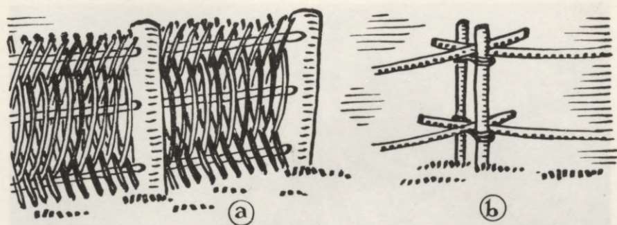
Sētu (žogu) veidi: zedeņu žogs (a); kāršu sēta (b).
