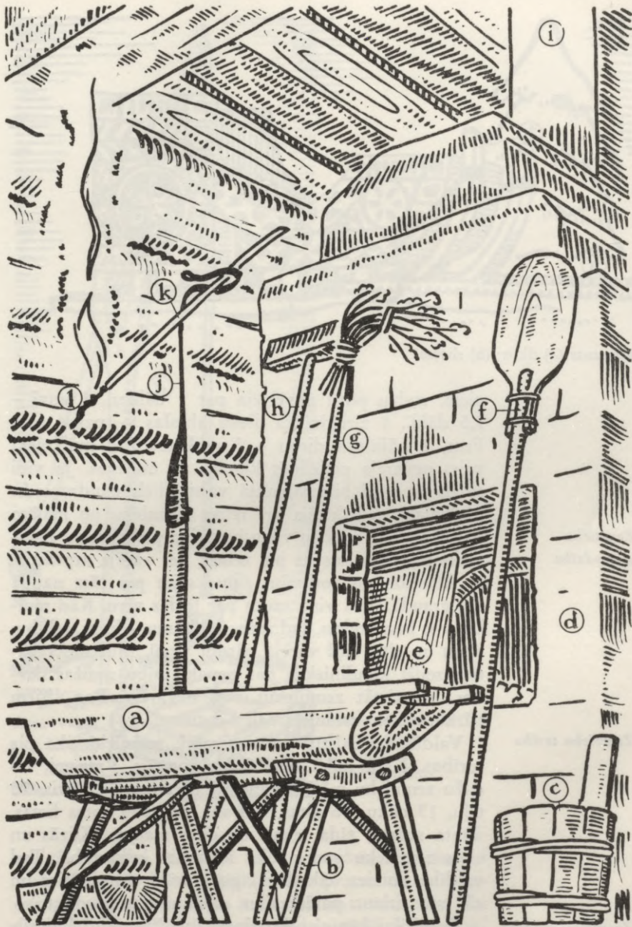
Maizes krāsns un abra a - abra; b - krāģis abras uzlikšanai; c - ķipsis; d - krāsns; e - krāsns plāte; f - lize; g - krāsns slota; h - krāsns kruķis; i - skurstenis; j - lākturis; k - skals; l - ogle.
