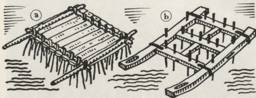
Koka ecēšas (a), darinātas no šķeltām zarainām egļu galotnēm, sastiprinot tās vienu otrai blakus ar zariem uz leju. Dzelzs tapu ecēšas (b) jaunākos laikos.
