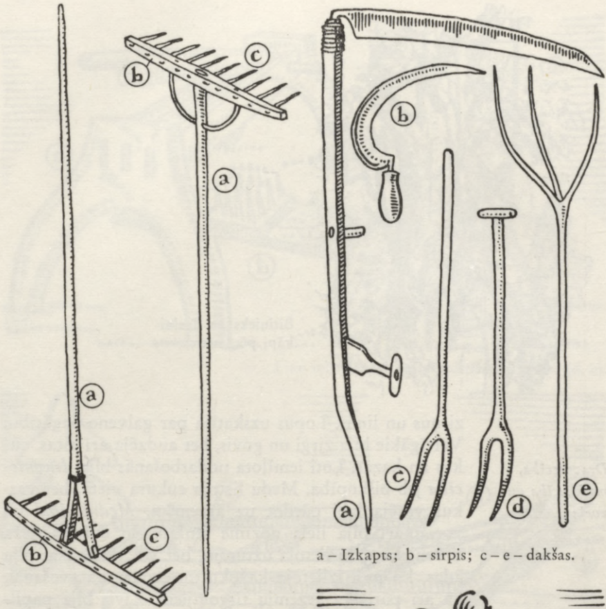
Grābekļi. a – Kāts; b – grābekļa galva; c – grābekļa zari.
