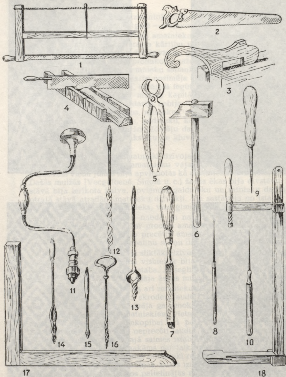
86. att. Lauku galdnieku darba rīki XX gs. sākumā:
