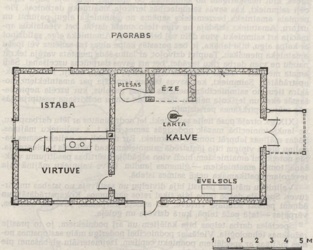
87. att. Lauku kalve XX gs. sākumā, Madonā.
