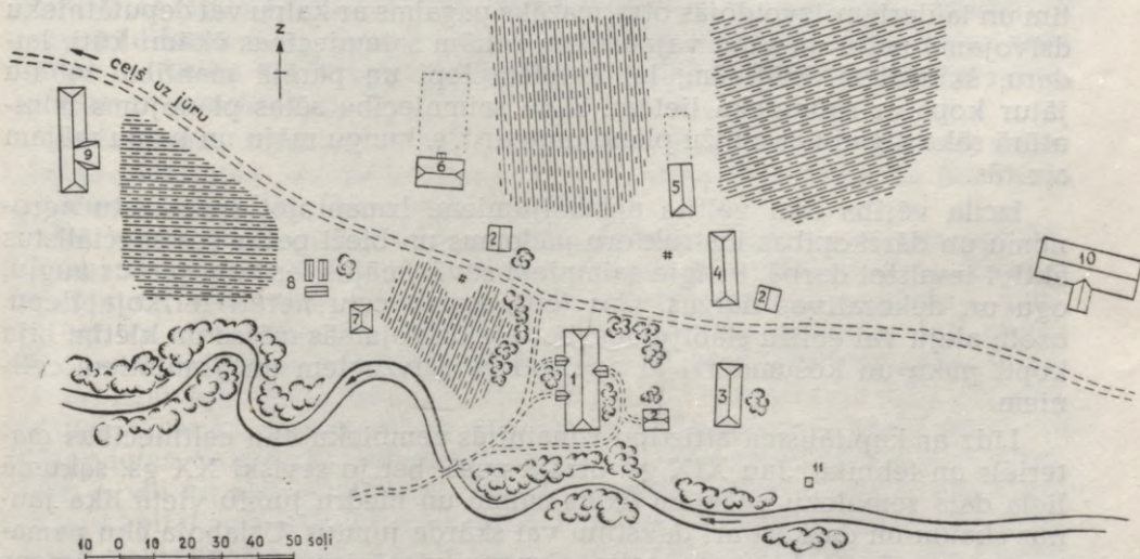
96. att. Turīgā zemnieka — zvejnieka dzīvojamā māja, celta ap 1900. gadu Vitrupē. Augšā ēkas ieejas fasāde no pagalma puses. Vidū — plāna shēma: 1 — kalpu dzīvojamā istaba; 2 — kalpu virtuve; 3 — pieliekamais; 4 — saimnieka virtuve; 5 — saimnieka dzīvojamās istabas; 6, 7 — bijuši saimnieka viesistaba — zāle, no kuras tagad atdalīta virtuve (6); 8 — veranda; 9 — lievenis. Apakšā: pagalma situācijas plāna shēma: 1 — dzīvojamā māja; 2 — klēts; 3 — trīsdalu klēts; 4 — jaunā kūts; 5 — vecā kūts; 6 — vecā dzīvojamā rija ar piedarbu (vēlāk kalpu māja); 7 — pirts; 8 — sakņu pagrabi; 9 — rija; 10 — šķūnis; 11 — ateja. 20 — Latviešu etnogrāfija
