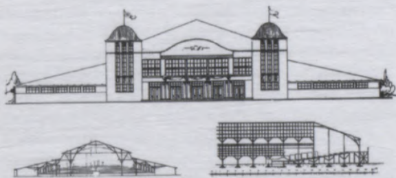
E.Poles projekts V Vispārējo dziesmu svētku halles celtniecībai Rīgā 1910. gadā.
