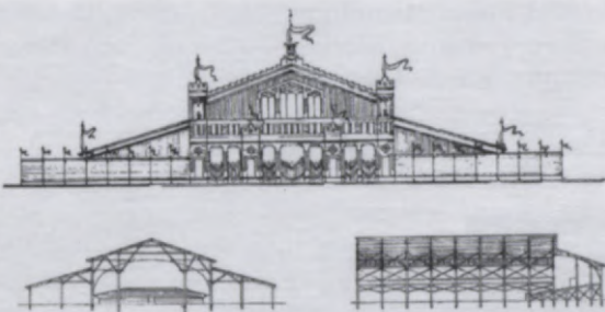
J.F.Baumaņa projekts II Vispārējo dziesmu svētku halles celtni 1880. gadā.
