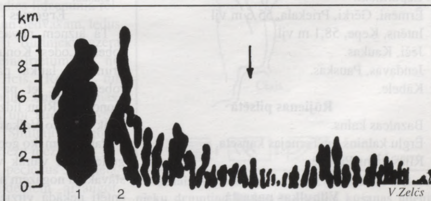
Drumlinu izmēri Rūjienas apkārtnē. 1 - Koņu kalns, 2 - Sedvakas kalns
