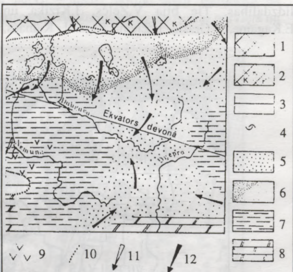
Baltijas devona paleogrāfiskā shēma
