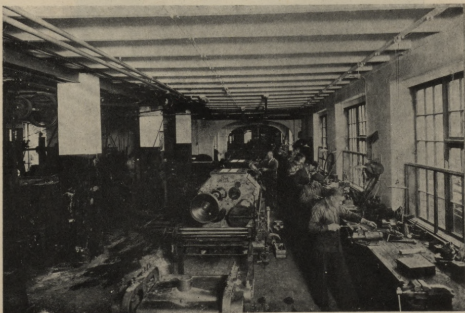
Plašu lomu spēlē mūsu fabrikas produkcijā dzirnavu mašīnu izgatavošana un sevišķi pēdējā laikā ienākuši daudz pasūtījumi valču krēsliem. Attēlā redzam dažus valču krēslus gatavošanā.
