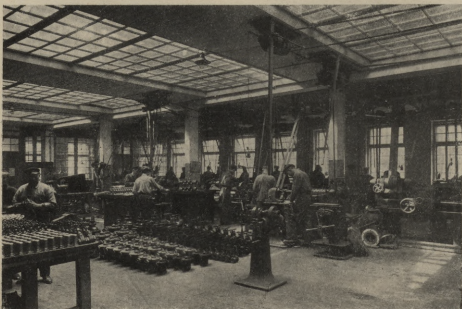
Atlējumi pēc tīrīšanas nokļūst plašā armatūru darbnīcā, kurā darbojās liels skaits virpmašīnu un speciālmašīnu.
