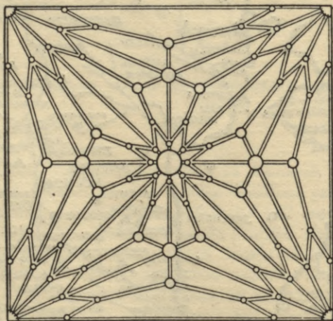
Cēsu pils Ordeņa mestra telpas velvju sistema.
