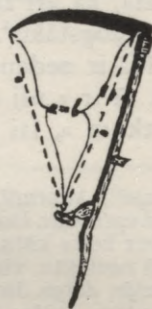
35. att. Izkaptis ir kņuba, ja asmens smailais gals ir no kūliša taisnā līnijā (a) tikpat tālu kā asmens platā gala stūris (b). Stendē. (Autora zīm.)
