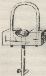
160. att. Koka grizeklis, ko uzmauc uz zirga mietiņa, lai nesapiņķējas virvē. Sakā. (Bīlenšteins.)
