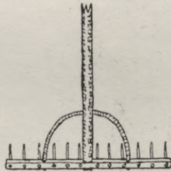
40. att. Grābekļa kāts ielaists tieši siekstā, un savienojums nostiprināts vēl ar saliektu kociņu, kas izvērts caurī kātam un siekstai. (Autora zīm.)
