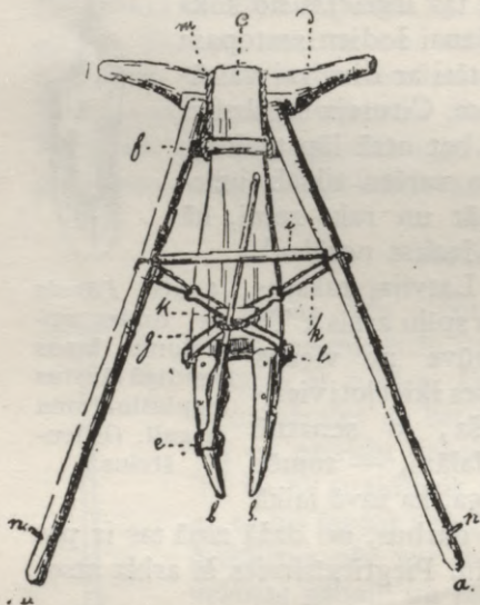
6. att. Spīļu arklis . (Bīlenšteins.) aa) apīžas, bb) lemeši, c) lemesnīca, d) balsts, e) vērstava, f) skalbīš jeb virsauklis, g) gredzeni jeb spandas, h) spandū auklas, i) sprūds, k) sprūdiņš jeb «dvēzele», l) apakšējais auklis, m) balsta auklas, nn) ilksu pulkas jeb «apīžas zari».
