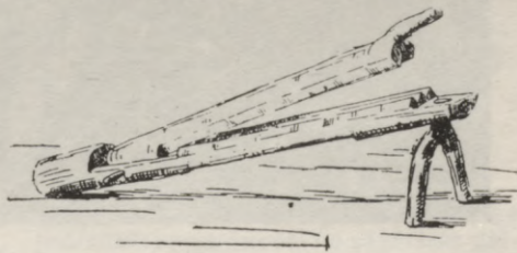
100. att. Mīstīklas . To kājas ieliktas no cita divzaraina koka. (Bilenšteins.)
