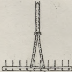
39. att. Grābekļa kāta resgalis iešķelts un tā zāķles gali iestiprināti siekstā un no otras puses vēl noķīlēti. (Autora zīm.)
