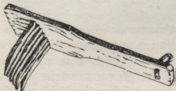
91. att. Vaļīgā suka — plese. (Vārsbergs.)
