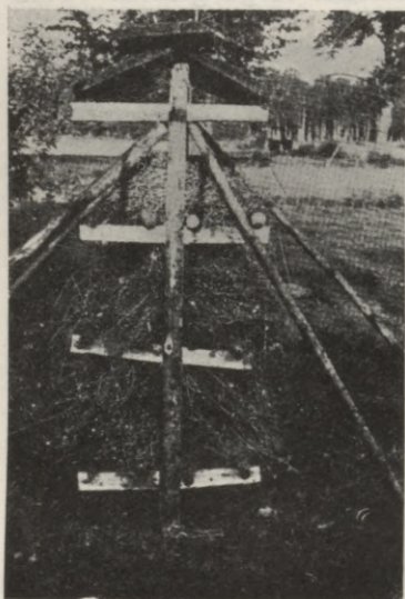
95. att. Tas pats žeperis pogaļu zeģināšanai. Skats no gala. Valgundē, 1936. g. (Autora uzņ.)
