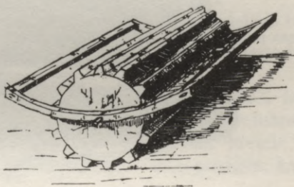
70. att. Rievainais veltenis. (Bilenšteins.) Kūlenis ir no smaga koka, apm. 4 pēdas gaŗš un 53 cm resns. Latas izcirstas no bērza vai oŗa koka; tās ir 8 cm platas un tikpat augstas. Laņķertu garenie koki ir 115 cm gaŗi, to likie sānkoki — 97 cm.
