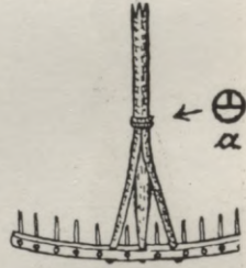
41. att. Dubultkāts ar divreiz pāršķeltu zāķli. Sieksta mazliet izliekta, lai labāk aptvertu sacirsto siena klēpi. (Autora zīm.)
