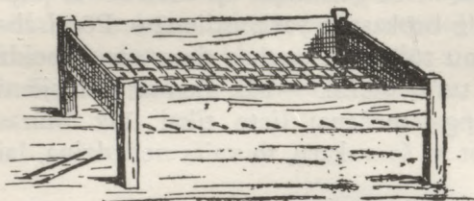
73. att. Režģu siets jeb kratīklas salmu kretelēšanai. (Bilenšteins.)
