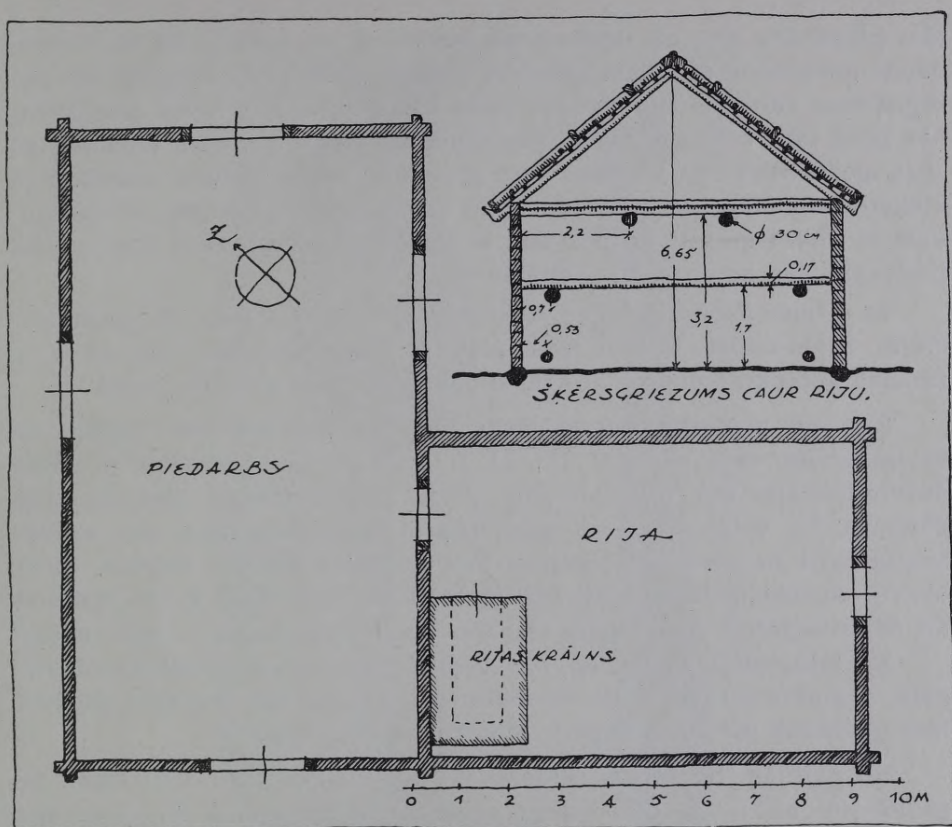
24. zīm. Rija. Kuldīgas apr. Rendas pag. „Mazputniņu” mājās.
