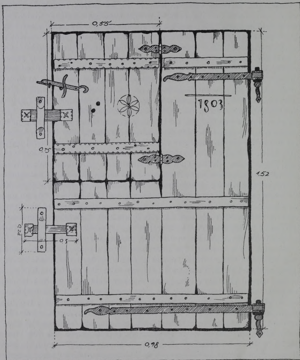
10. zīm. Istabas ārdurvis. Liepājas apr. Rucavas pag. Papes ciemā.
