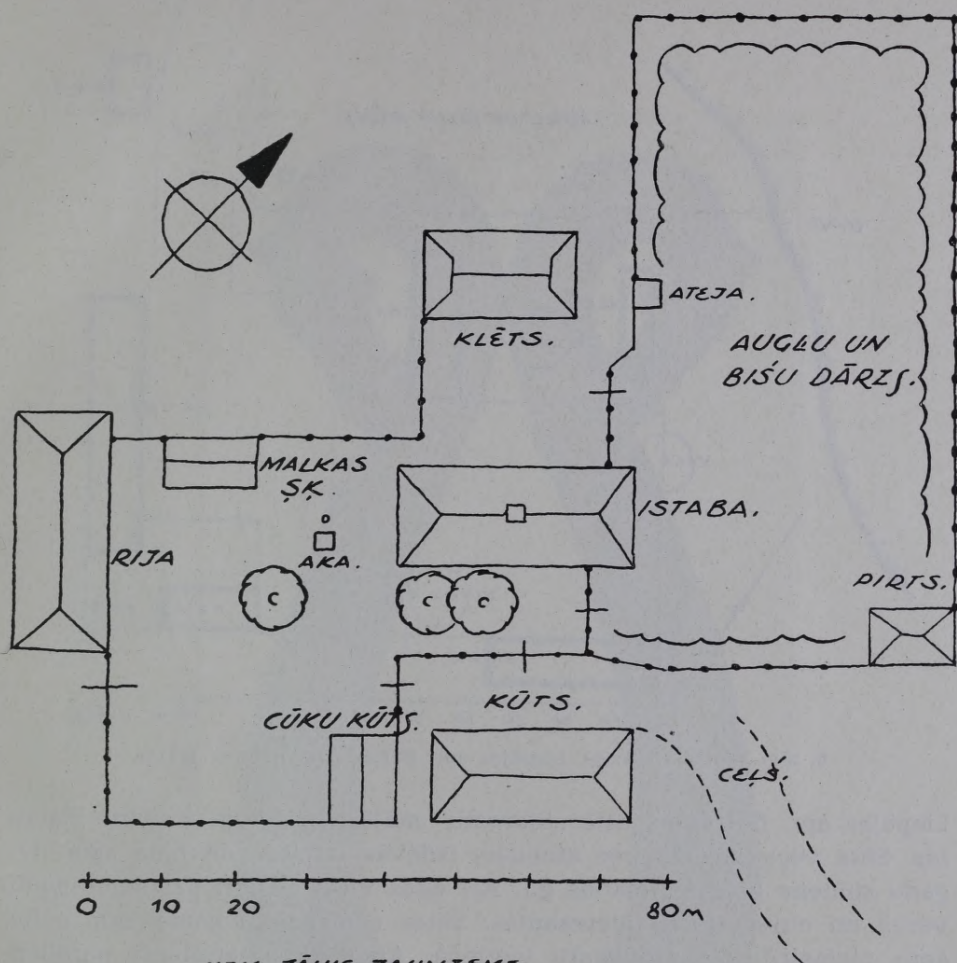
5. zīm. Sētas situācijas plāns. Liepājas apr. Bārtas pag. „Starostu” mājās.
