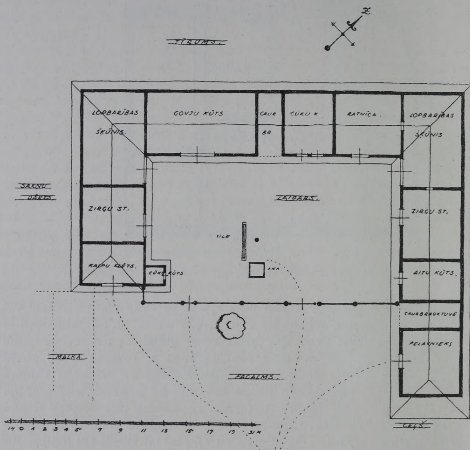
22. zīm. Kurzemes „dīzais laids”. Liepājas apr. Rucavas pag. „Deju” mājās (tagad Brīvdabas mūzejā).
