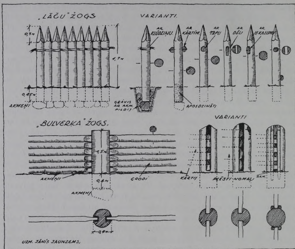
8. zīm. Žogu veidi Kurzemē.
