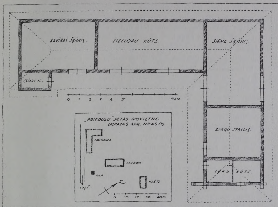
23. zīm. „Dižais laidars”. Liepājas apr. Nīcas pag. „Priekuļu” mājās.
