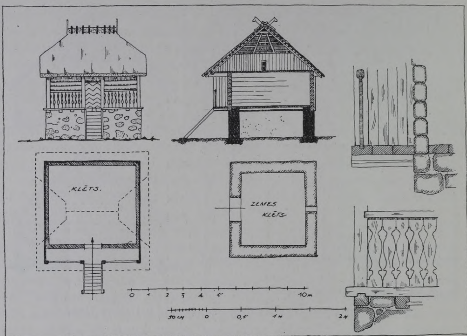
18. zīm. Klēts. Liepājas apr. Nicas pag. „Jaunzemju” mājās.
