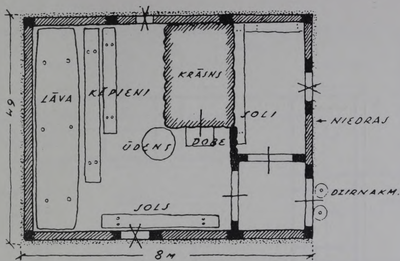
21. zīm. Pirts plāns, Liepājas apr. Nīcas pag. „Spirēnos”.
