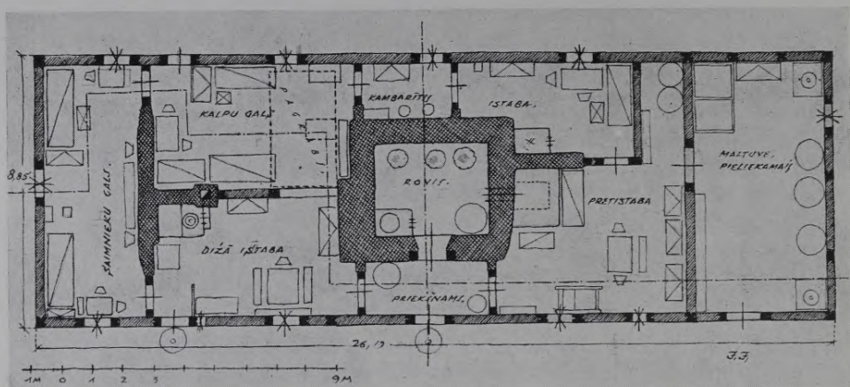
13. zīm. Dzīvojamās ēkas plāns. Kuldīgas apr. Snēpeles pag. „Laucinieku” mājās.
