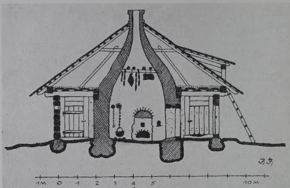
15. zīm. Dzīvojamās ēkas konstruktīvs šķērsgriezums. Kuldīgas apr. Snēpeles pag. „Laucinieku” mājās.
