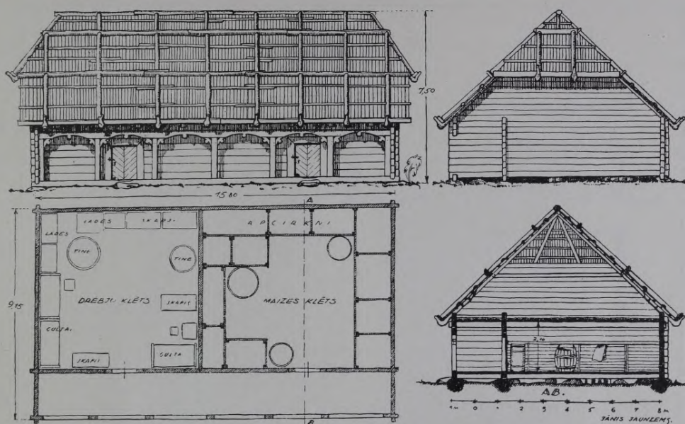
17. zīm. Klēts uzmērījums. Kuldīgas apr. Rendas pag. Apes ciemā.
