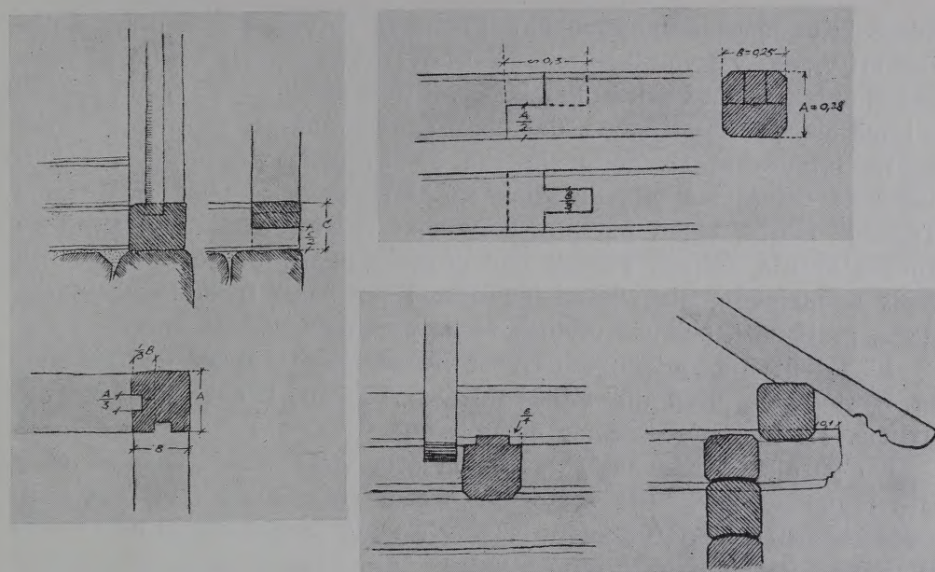
16. zīm. Konstruktiņas sīkdaļas dzīvojamai ēkai. Kuldīgas apr. Snēpeles pag. „Laucinieku” mājās.
