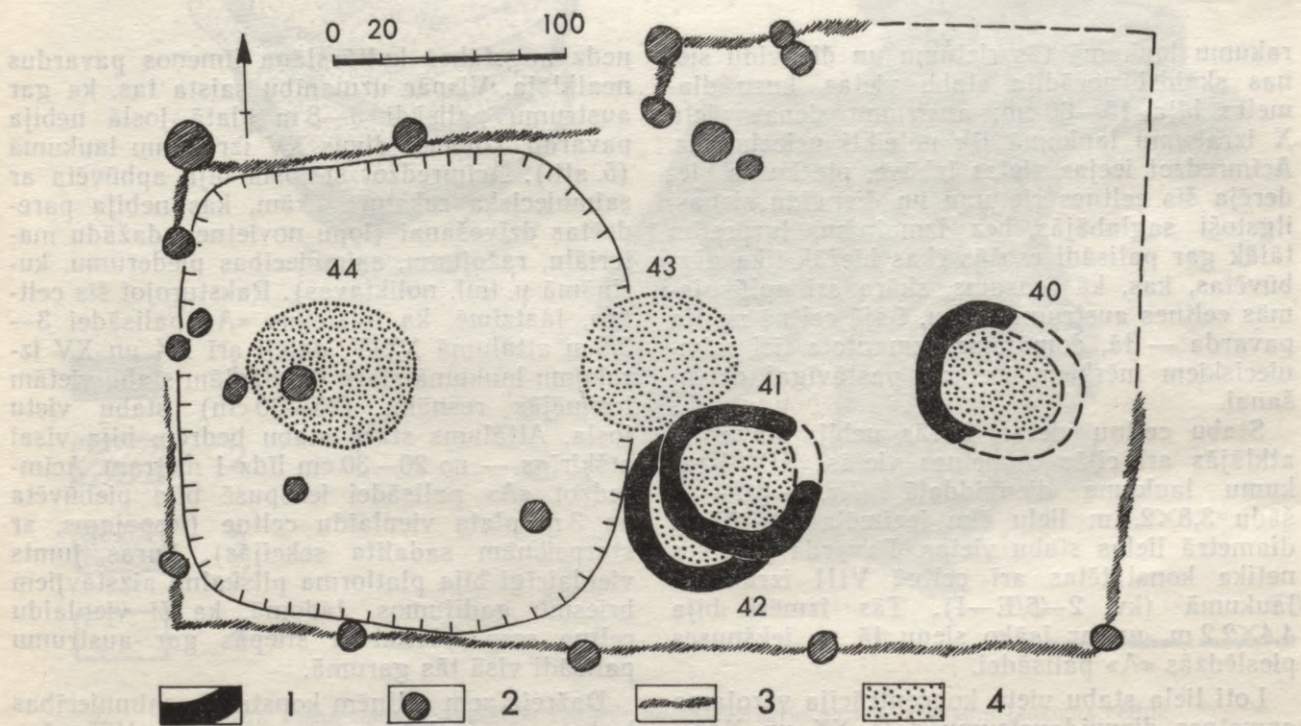
24. att. Celtnes vieta XVIII izrakumu laukumā.
