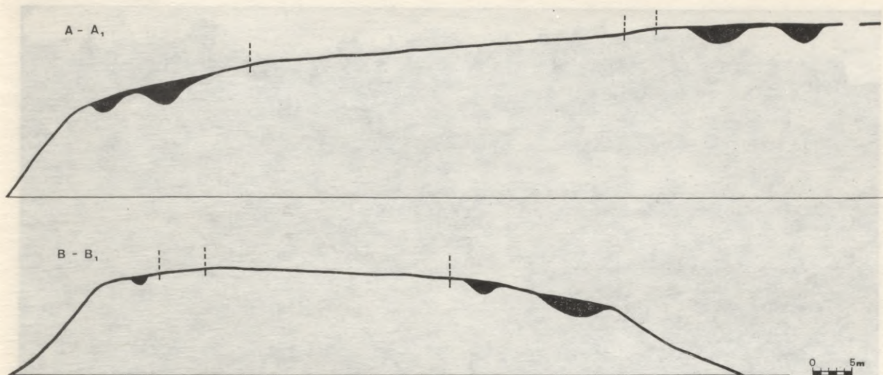
6. att. Brikūļu nocietinātās apmetnes šķersgriezums pa A—A 1 un B—B 1 (sk. 5. att.). Cross-section of Brikūļu fortified settlement along A—A 1 and B—B 1 (see fig. 5).
