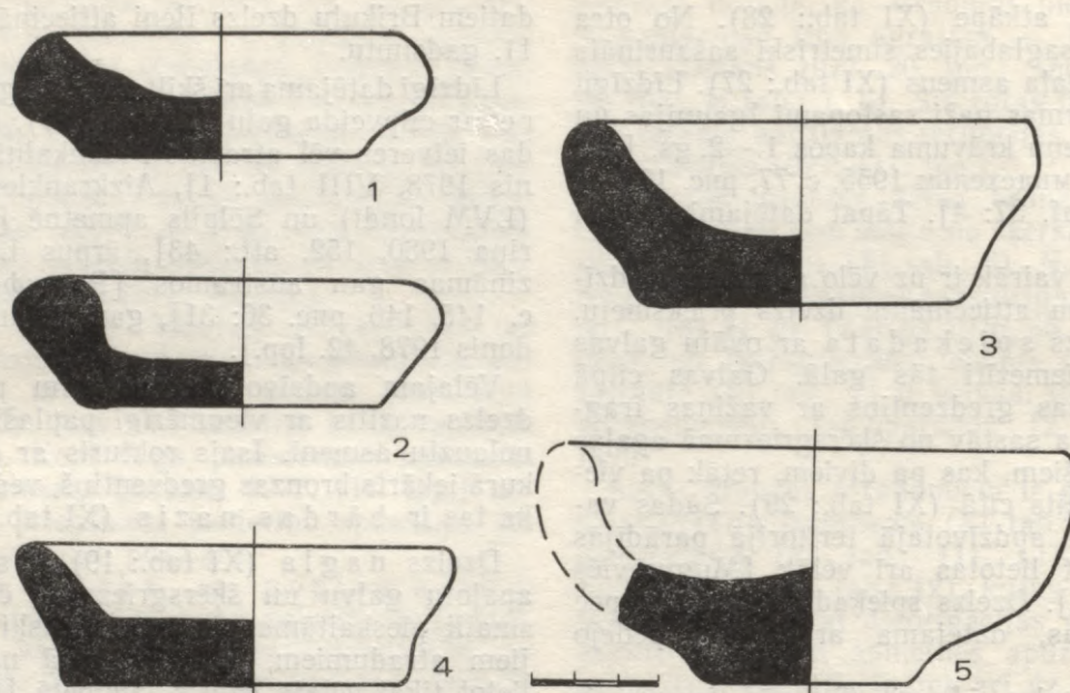
33. att. Māla tīģeļu formas.
