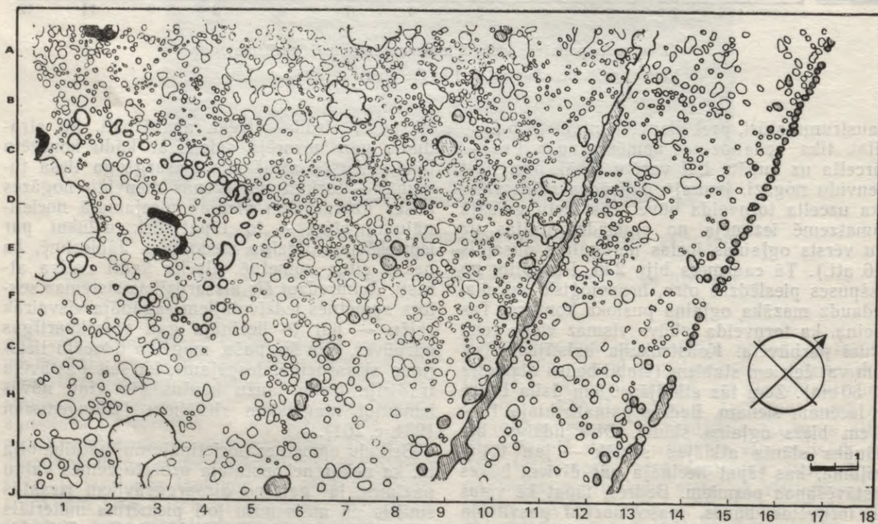
13. att. «A» un «B» palisādes vieta XXIV izrakumu laukumā. Palisāžu norobežotajā plakuma daļā gaišā pamatzeme bija izraibināta ar mietu un stabu vietām, kas liecināja par stabu konstrukcijās celto ēku blīvo izvietojumu un pārbūvēm.
