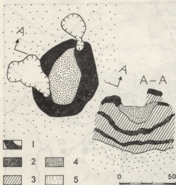
21. att. Pavardi nr. 11—14 iedziļinātā celtnē V izrakumu laukumā. Šķērsgriezumā A—A divi apakšējie kloni pieder pavardiem bez māla apmales; virs tiem divi pavardi ar māla apmali.
