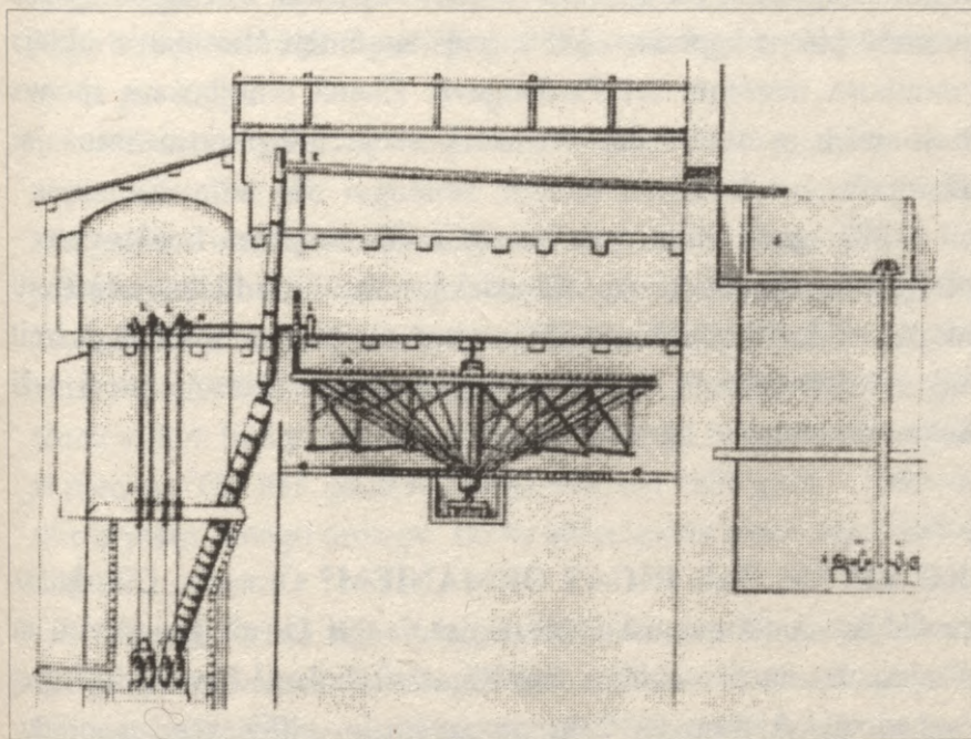
Ūdens apgādes ierīce Zunderna tornī (19. gs. pirmā puse)
