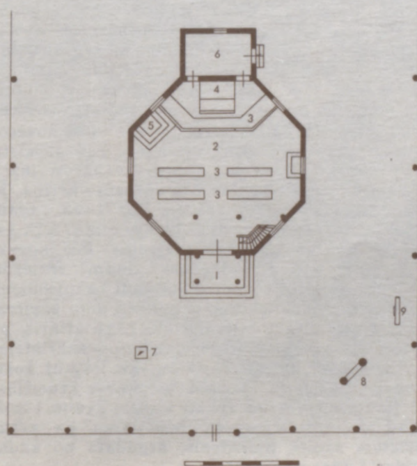
Daugavpils, Rudzātu Eleonorvīles katoļu kapelas plāna shēma:
