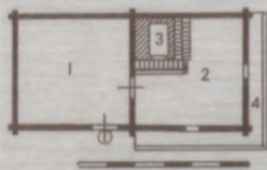
Rēzekne, Gaigalavas Meirānu dūmistabas plāna shēma:
