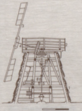
Rēzekne, Dricēnu Der- vinieku vējdzirnavu patmaļu griezuma shēma:
