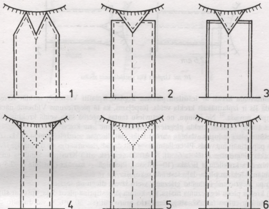
7. att. Uzpleča ķīļa iestrādes varianti
