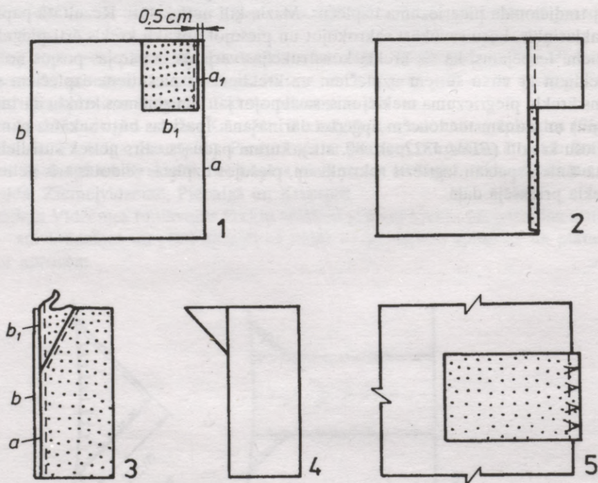
13. att. Tunikveida krekla ar iešūtiem pleciem piegrieztne
