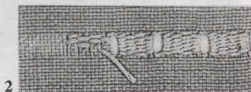
50. att. Caurā vile
