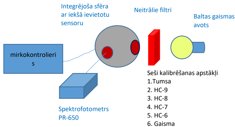
3. att. Sensoru kalibrēšanas procesā iesastīta aprīkojuma shēma. Sensori ir ievietoti integrējošā sfērā un pasargāti no tiešajiem stariem ar aizsegu, tā lai tvertu tikai vienmērīgi izkliedētu gaismu.
