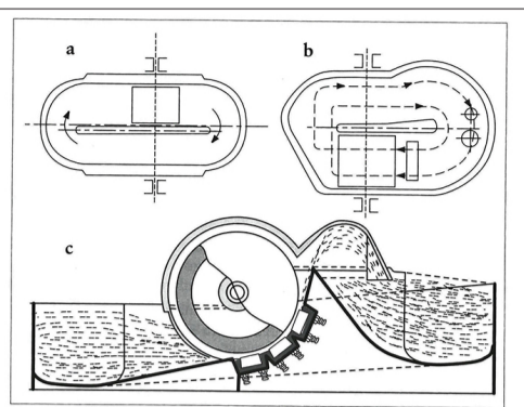
14. attēls. Holendera shēma (virskāla) masas plūsmas: a – holendera vannā ar ovāliem galiem; b – holendera vannā ar speciāli izveidotu galu, masas labākai maisīšanai. c – Holendera shēma (sānskatā). 1 – holendera vannas; 2 – rotējošs mašīnas veltnis ar nažiem, pamatnažu plankas; 4 – veltnu vāks; 5 – uzstājņi.
