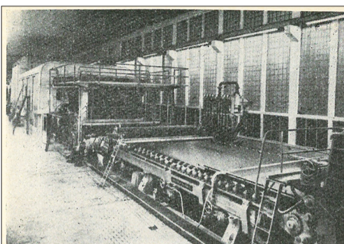
27. att. Moderna papīrmašīna no sieta galda puses.
