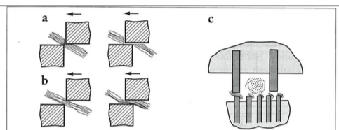
13. attēls. Mašīnas iekārtas nažu darbības shēma: a – šķiedras saīsināšana; b – šķiedras apļūnāšana; c – šķiedru kārtības veidošanās uz nažu malām.
