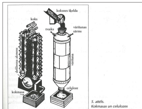
Koksmas uz celulozes iegūšanas shēma. No grāmatas V. Norīte, V. Turlais, D. Vanaga. Poligrāfija
