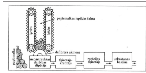
Baltās koksmas ražošanas shēma. No grāmatas V. Norīte, V. Turlais, D. Vanaga. Poligrāfija
