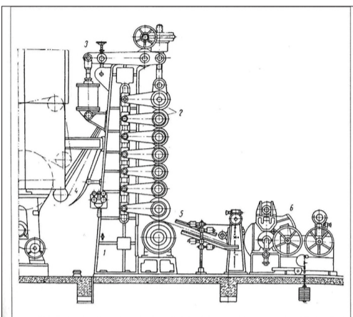
43. attēls. Mašīnkalandrs: 1 – stātnis; 2 – veltnis; 3 – pneimatiska veltnu pacelšanas un piespiešanas ierīce; 4 – papīra ievadīšana; 5 – papīra izvadīšana; 6 – uzstājņi.
