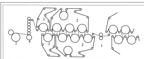
42. attēls. Papīrmašīnas noslēguma daļas shēma: 1 – sāpju kalandrs vai līmes prese; 2 – pedēja žāvēšanas grupa; 3 – dzesēšanas cilindrs; 4 – mašīnkalandrs; 5 – uzstājņi.
