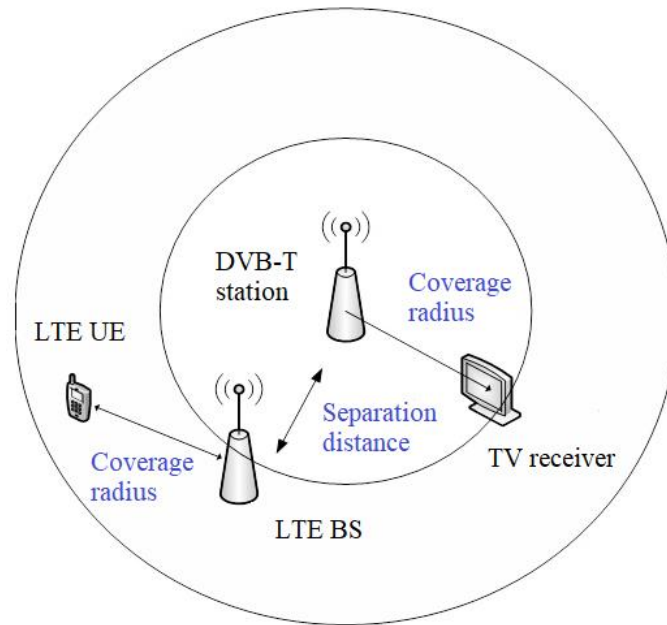
Fig. 3.1. SEAMCAT simulation scenario.
