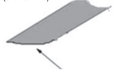
“Полукруглая” заточка, бур катится на “дуге” и не бурит (схематично).
