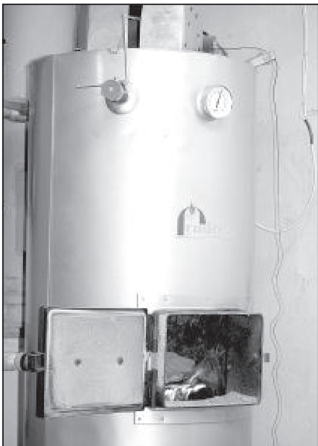
Этот котел отапливает помещения с помощью брикетов.
