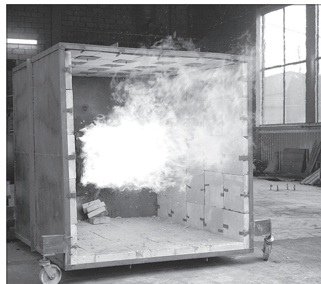
Горение газа в модели котла.
