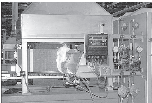
Печь для закалки металлических деталей в действии.
