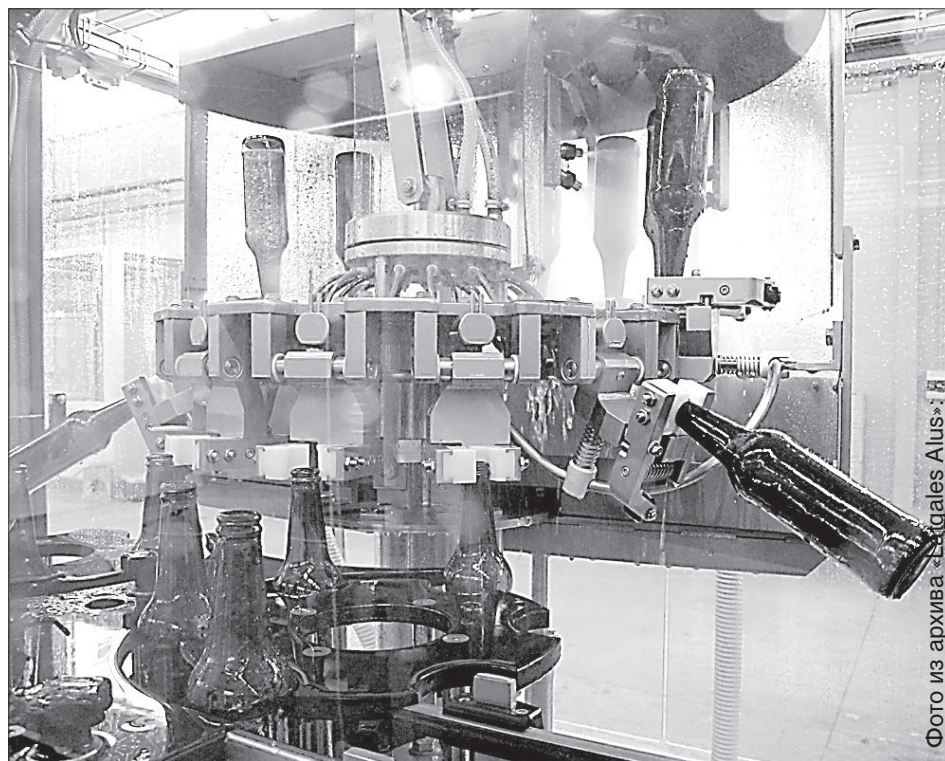
Мойка и сушка бутылок перед розливом.
