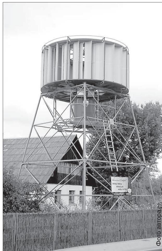
Ветряной генератор.
