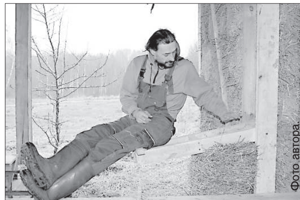
Оскар демонстрирует, как в стенах укрепляются соломенные колоды.
