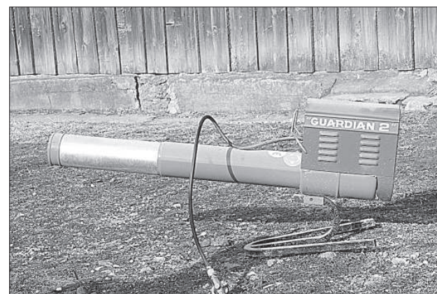
«Пушка» для отпугивания птиц.
