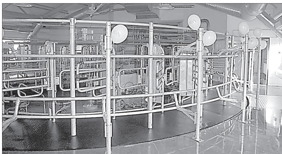
Доильная карусель.
